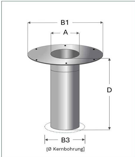
PVC-Hartflansch
