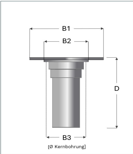
PVC-Hartflansch (Seitenansicht)
