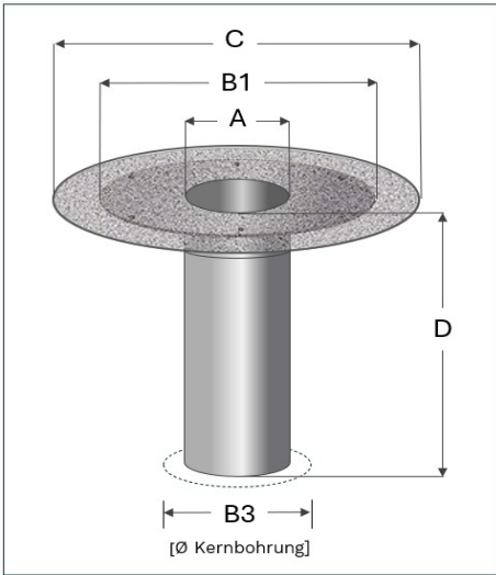
Bitumen-Manschette
