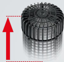
Die Idee: Ein Laubsieb, das sich bei 60 mm angestaumtem Wasser mechanisch hebt.
