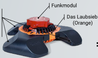
Der ROOFGUARD: Ein patentiertes Laubsieb mit Lift-Funktion und Funkmodul.
