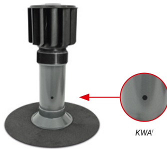
Im Bild: Flansch-Manschette aus Bitumen-Schweißbahn
