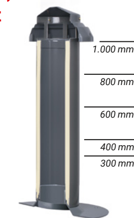
Schematische Darstellung
