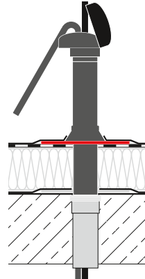
Im Bild: Flansch-Manschette aus Bitumen-Schweißbahn (Unterrohr abnehmbar)
