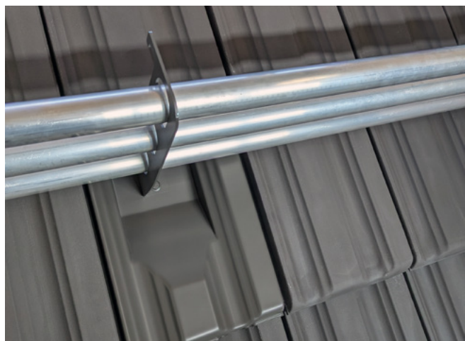
Kombi-Schneefangpfanne mit Rohren.
